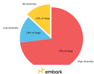
MHC Class II - DLA DRB1 No Diversity
